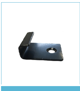
Starter inox galvanizzata nera per pezzi speciali WPC PROTECTA e WPC PROTECTA EVO (raccomandato 7 pz cadauno)
